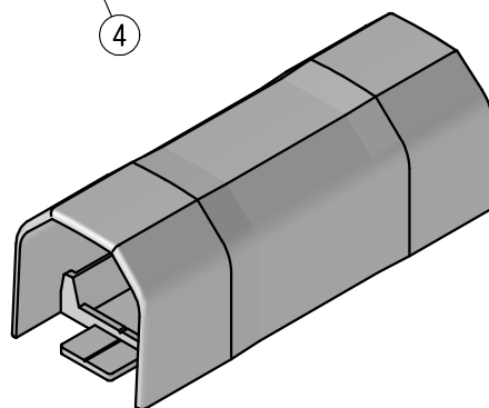
参考斜視図
